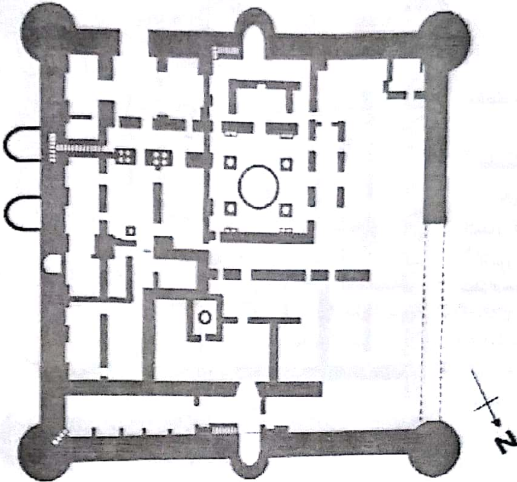
مخطط رقم (٣) مخطط قلعة بازيان البناء الأصلي - الدور الثاني مقياس الرسم (١ : ٢٠٠ سم)
