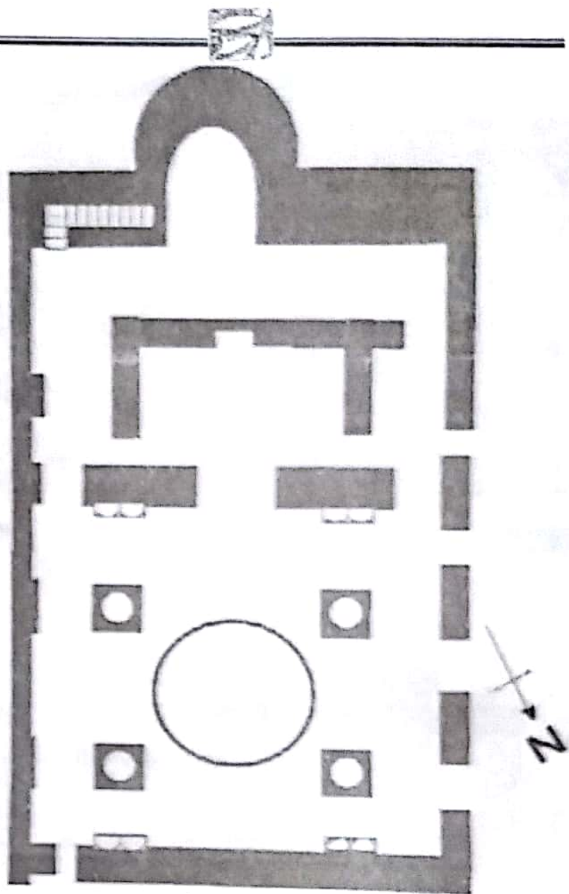
مخطط رقم (٧) جناح الوسط لقلعة بازيان - الدور الثاني - مقياس الرسم (١/٢٠٠ سم)
