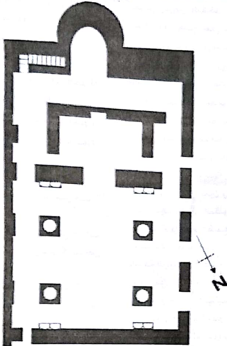
مخطط رقم (٦) جناح الوسط لقلعة بازيان - الدور الأول - مقياس الرسم (١ : ٢٠٠ سم)
